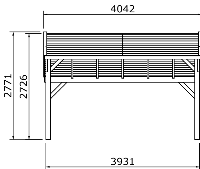
Vooraanzicht
