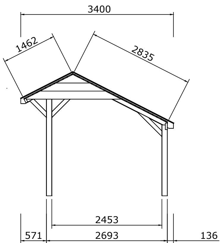
Rechter zijaanzicht
