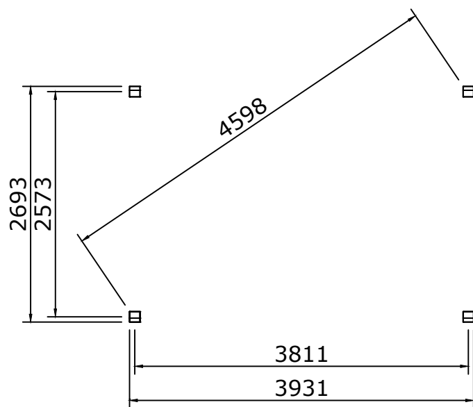
Palenplan
